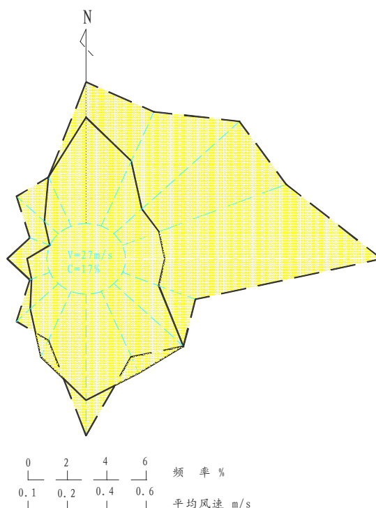
图 1.1 东莞市累年风向玫瑰图
